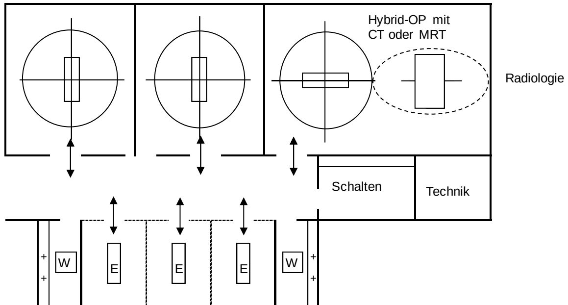
Abb. 28: Systemgrundriss Hybrid-OP mit CT
