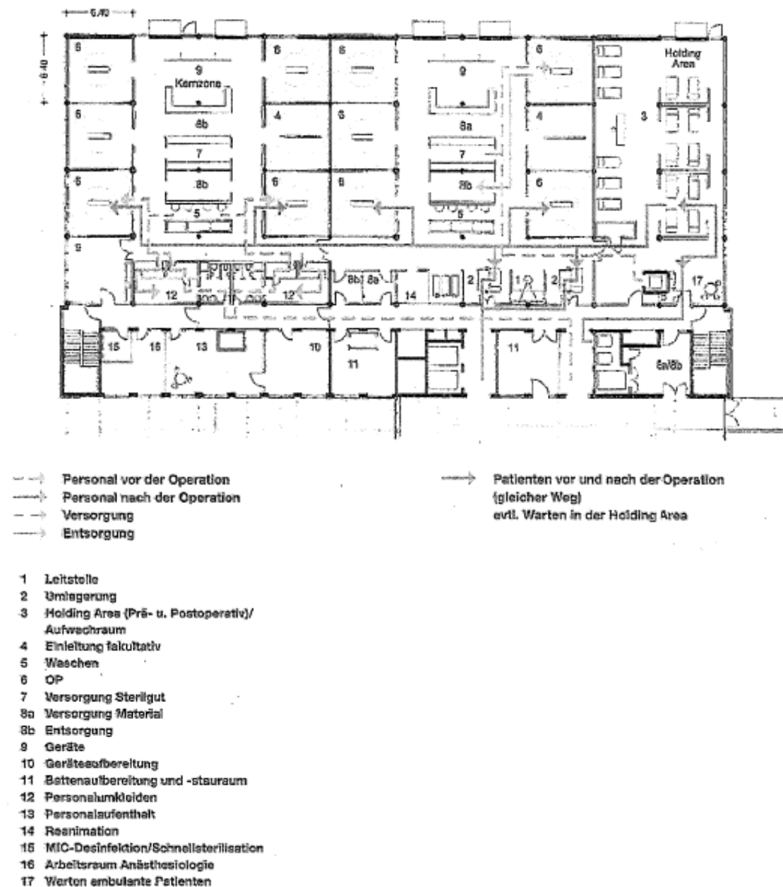
Abb 10: Städtisches Klinikum Brandenburg – OP-Abteilung (Arch: Heinle, Wischer und Partner, Berlin)
