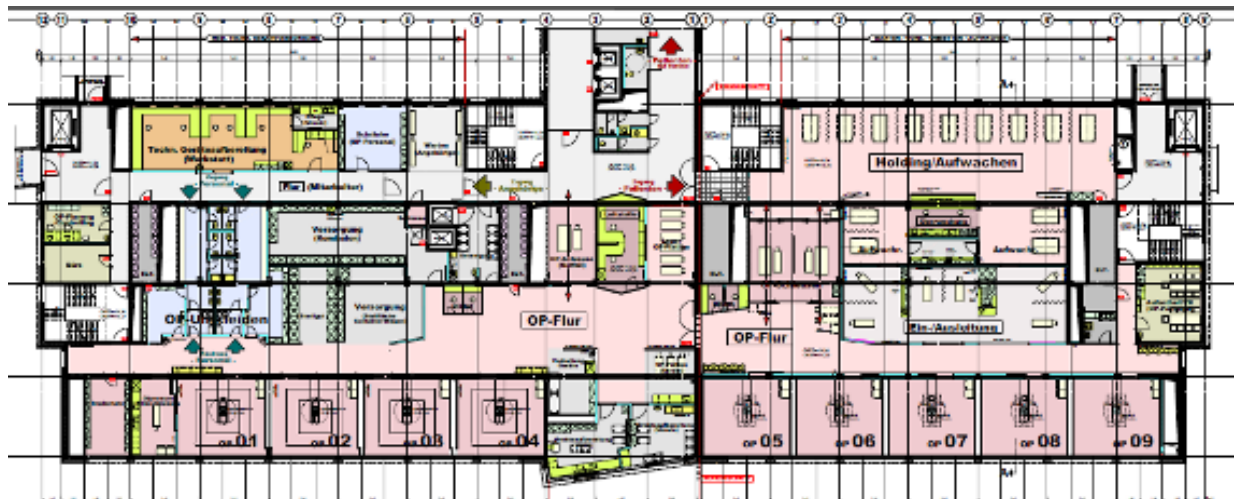
Abb. 11: Grundriss OP-Abteilung St. Bernward Krankenhaus Hildesheim, (Architekten Lohr und Lohr, Hannover)
